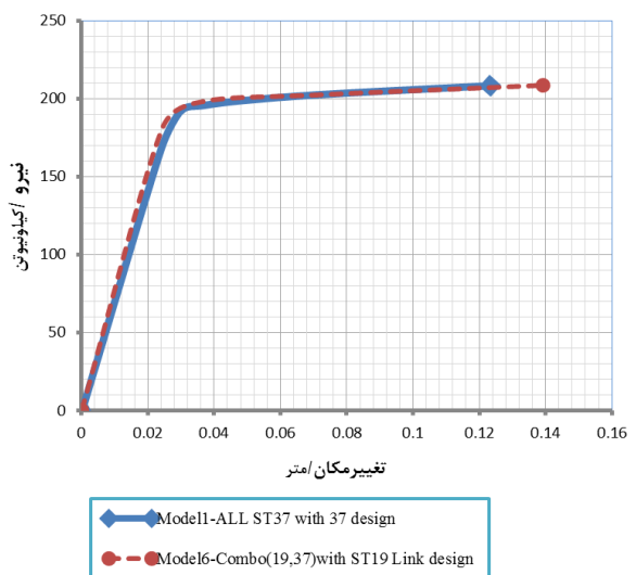
شکل (۱۱): مقایسه منحنی‌های پوش مدل‌های ۱ و ۶
